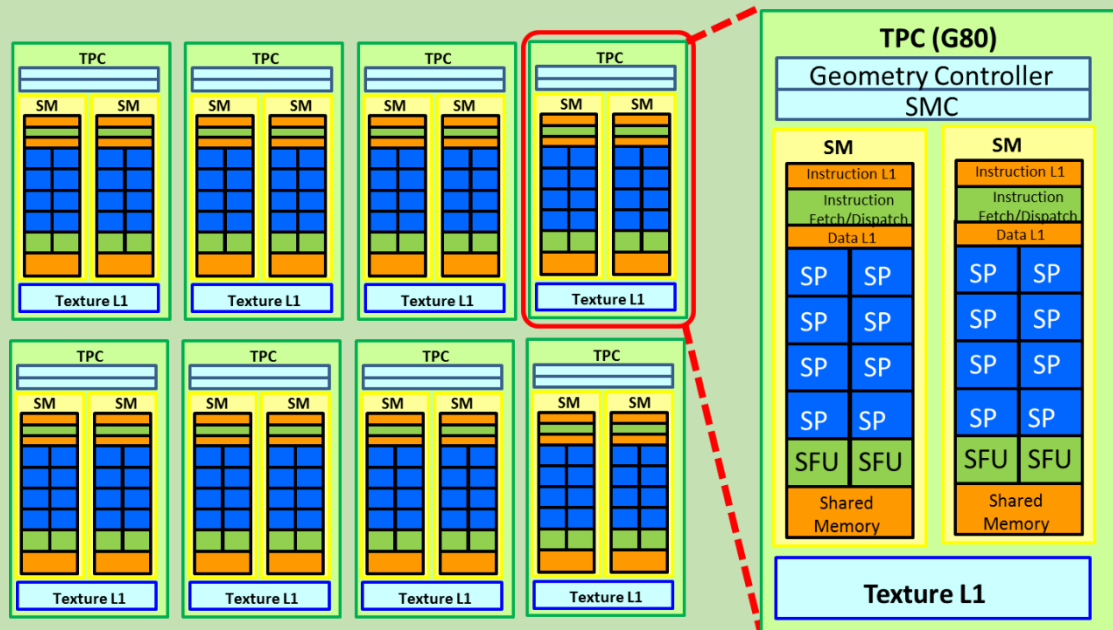
圖 2 NVIDIA G80 架構示意圖 ①
